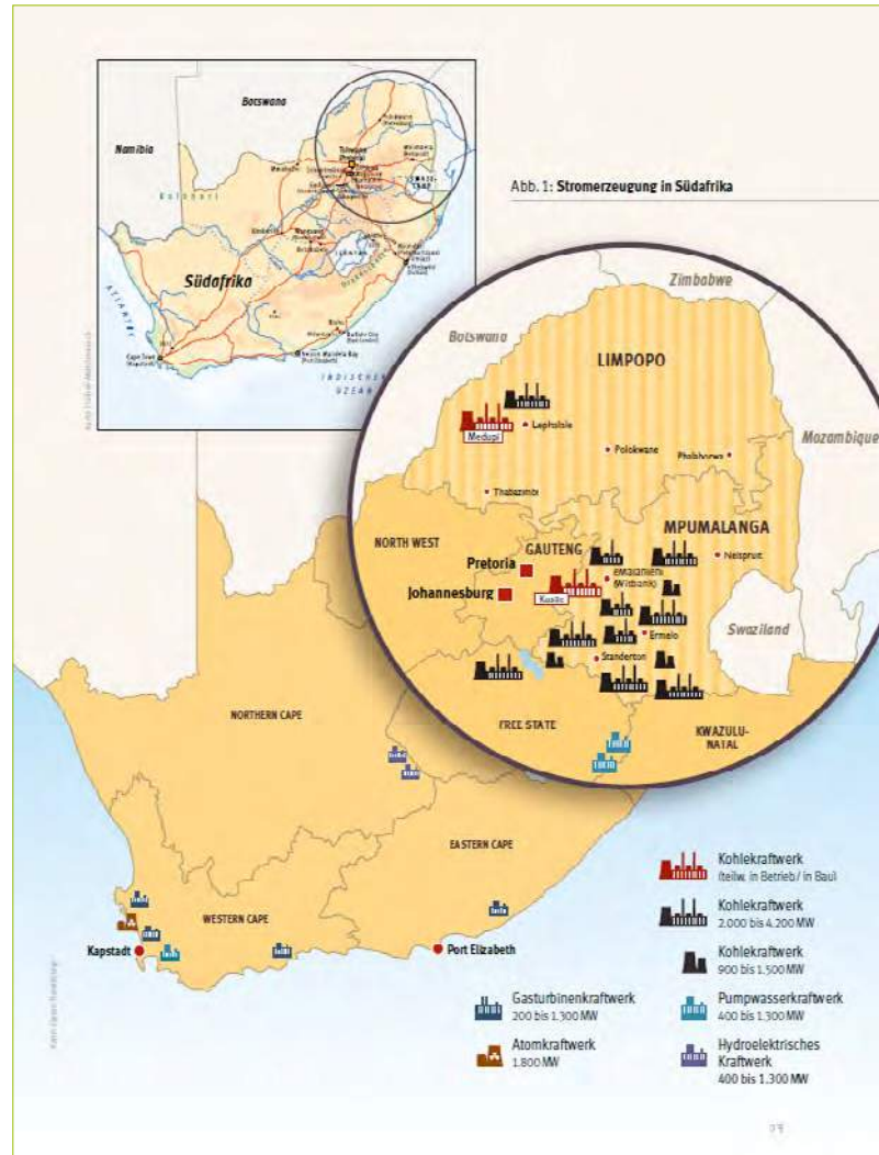
M21: Stromerzeugung in Südafrika (MISEREOR, 2015: Wenn nur die Kohle zählt, S. 23)
